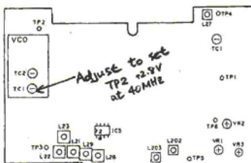
PLL UNIT (X50-3200-00)
