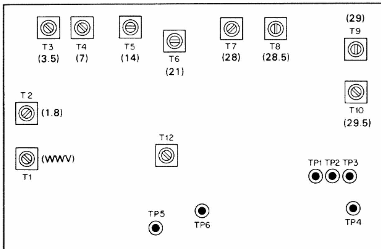
Fig. 22 VCO unit
